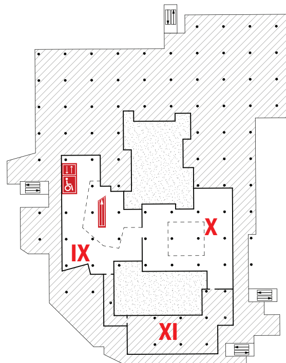
1 Untergeschoss
